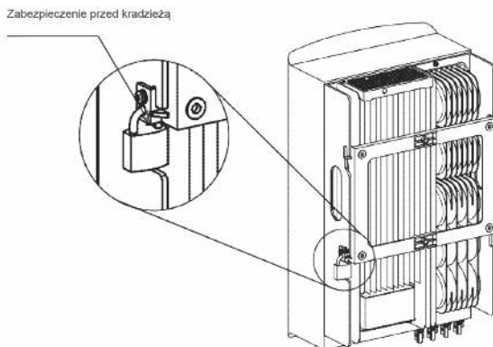
Rysunek 5.6 Mocowanie falownika
