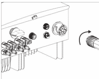
Rysunek 5.24 Złącze prądu przemiennego do falownika
