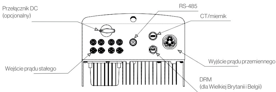
Rysunek 1.2 widok z dołu
