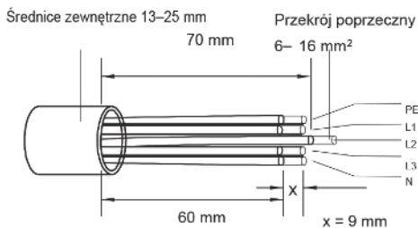
Rysunek 5.20 Przewód ze zdjętą izolacją i odsonięty
