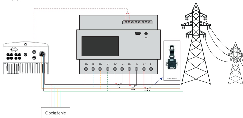
Rysunek 5.27 Podłączenie miernika (2)
