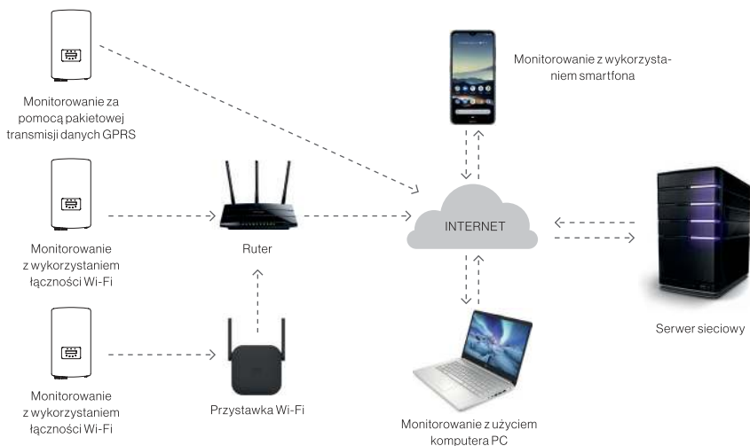
Rysunek 5.25 Funkcja komunikacji bezprzewodowej
