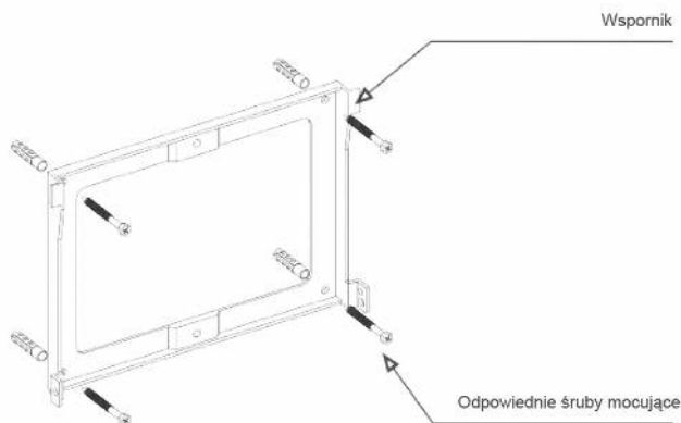
Rysunek 5.4 Montaż falownika na ścianie
