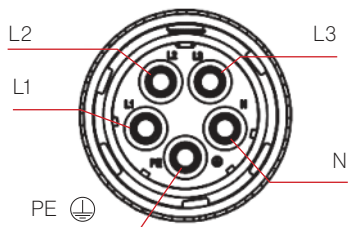
Rysunek 5.21 Konstrukcja wewnętrzna złącza prądu zmiennego
