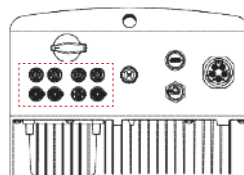
Rysunek 5.18 Podłączenie złącza prądu stałego do falownika
