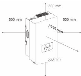
Rysunek 5.2 Obszar pomiędzy falownikiem a sąsiadującymi urządzeniami podczas montażu
