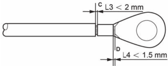
Rysunek 5.9 Przewód ze zdjętą izolacją
