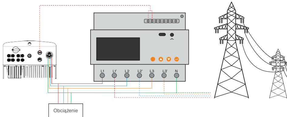
Rysunek 5.26 Podłączenie miernika (1)
