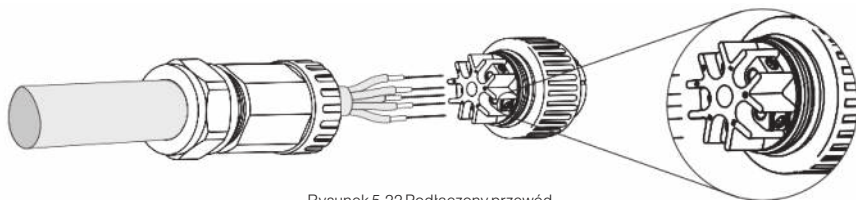
Rysunek 5.22 Podłączony przewód
