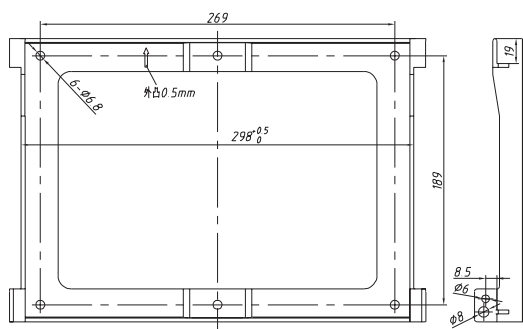
Rysunek 5.3 Montaż falownika na ścianie
